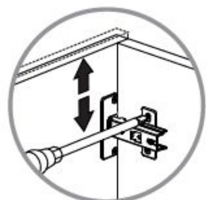
AJUSTE DE ALTURA / HEIGHT ADJUSTMENT
