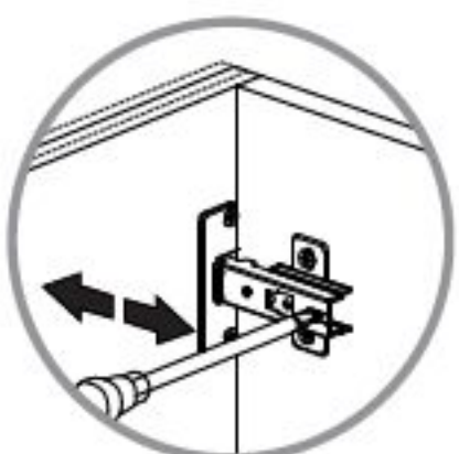
AJUSTE DE PROFUNDIDAD / DEPTH ADJUSTMENT
