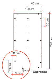
Montaje con tornillos.
