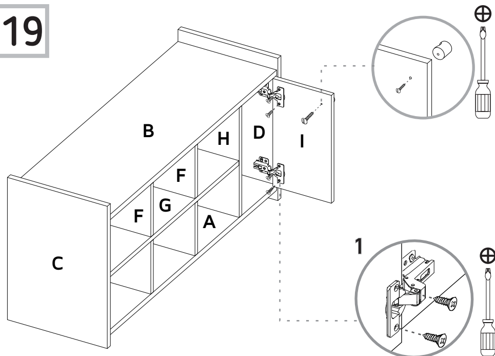
1 Ajuste de las bisagras Hinge adjustment
