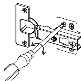
Ajuste tornillos frontales Front screws adjustment/ Réglage des vis avant
