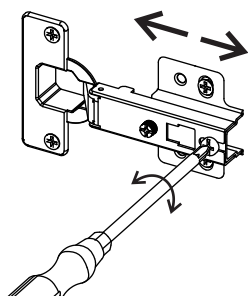
Ajuste de profundidad Depth adjustment/ Ajustement de la profondeur
