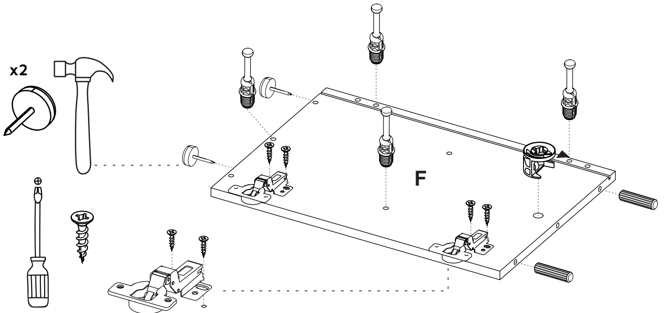
Instalación Bisagra Hinge installation / Pose de charnière
