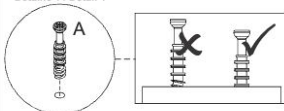
Detalle 1 / Detail 1 Detalhe 1 / Détail 1
