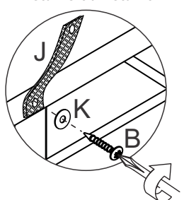
Detalle 6 / Detail 6 Detalhe 6 / Détail 6
