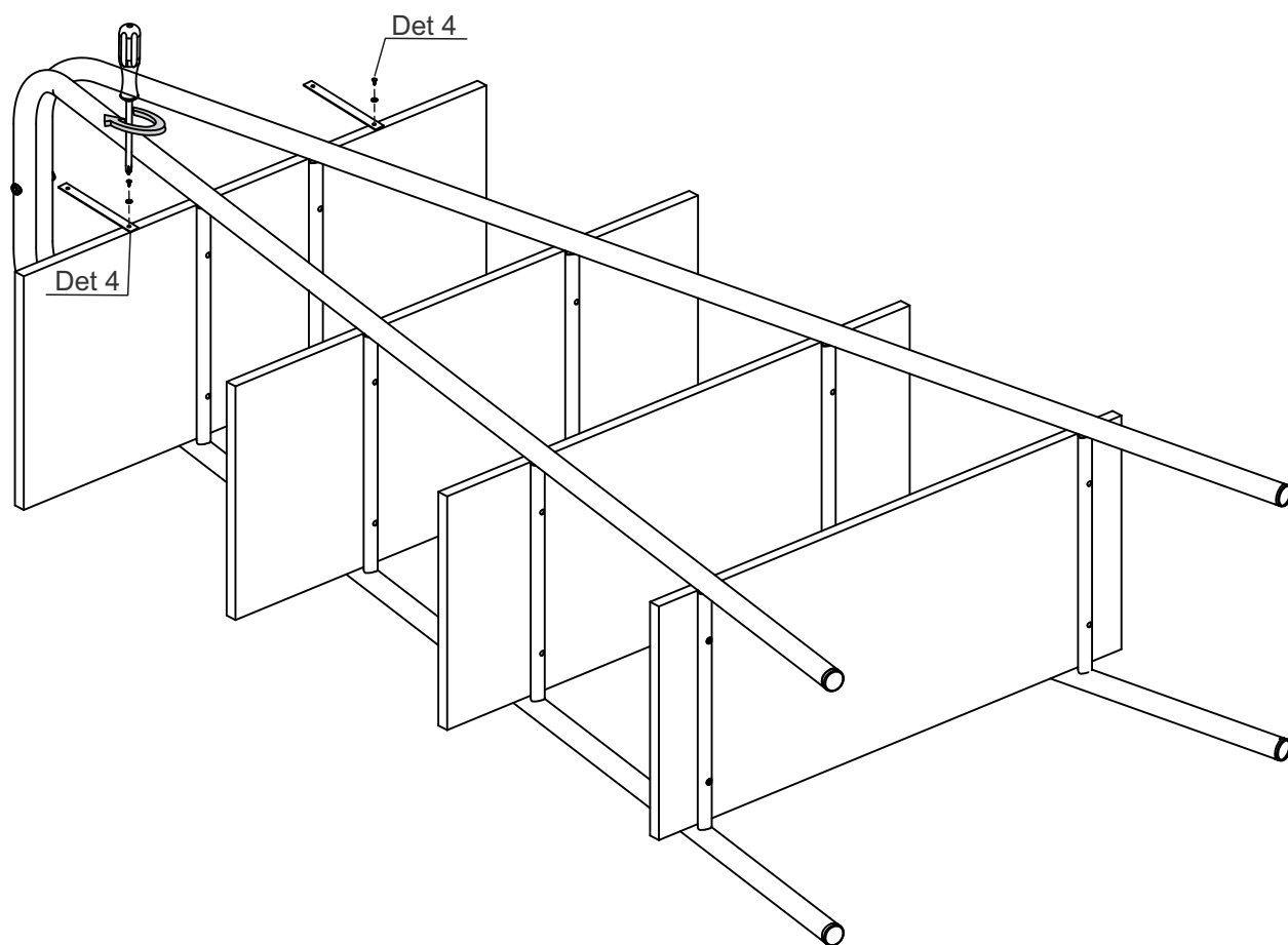
Detalle 4 / Detail 4 Detalhe 4 / Détail 4
