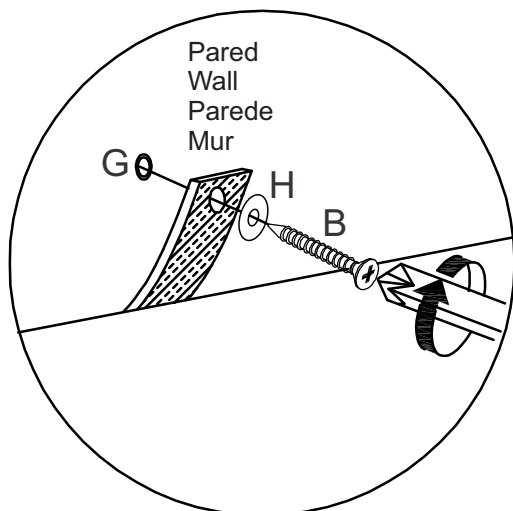
Detalle 6 / Detail 6 Detalhe 6 / Détail 6
