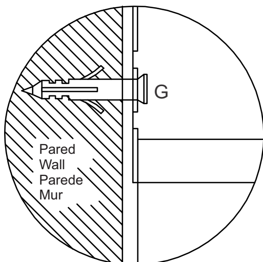
Detalle 5 / Detail 5 Detalhe 5 / Détail 5
