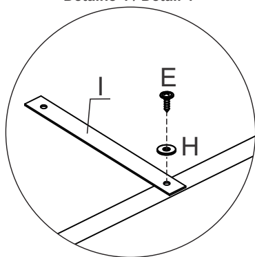
Detalle 4 / Detail 4 Detalhe 4 / Détail 4
