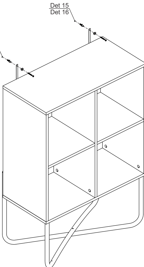
Det 15 Det 16
