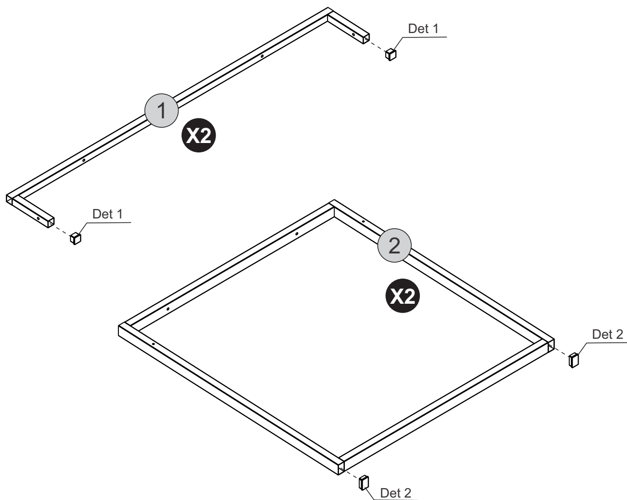
Detalle 1 / Detail 1 Detalhe 1 / Détail 1
